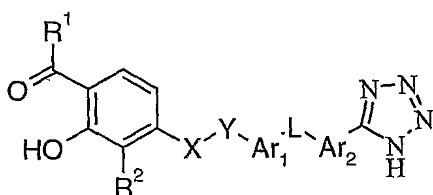
tautomer I
