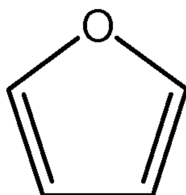
furyl
