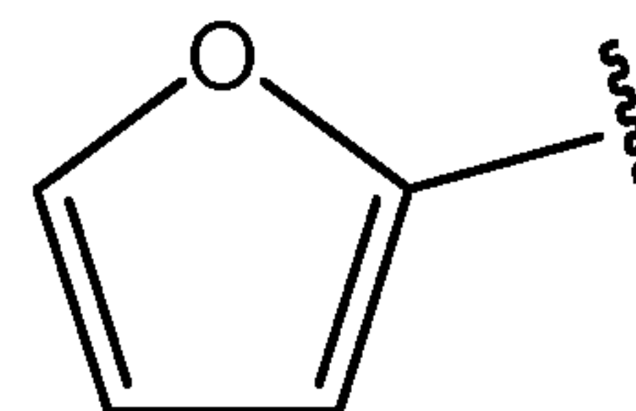
fur-2-yl
