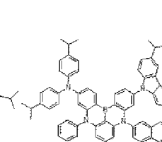
Dopant 115
