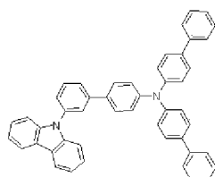
H17
