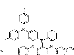
Dopant 88
