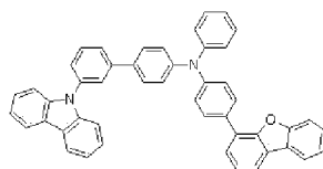
H22
