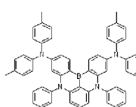
Dopant 58
