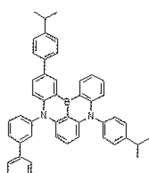
Dopant 44
