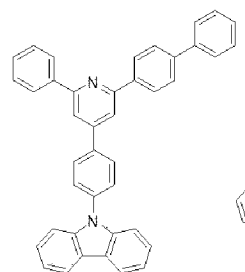
E10
