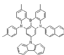
Dopant 98
