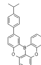
Dopant 180
