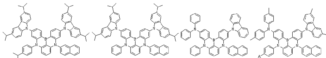
Dopant 109
