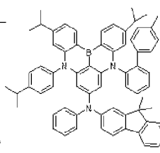
Dopant 131
