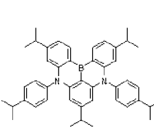
Dopant 139
