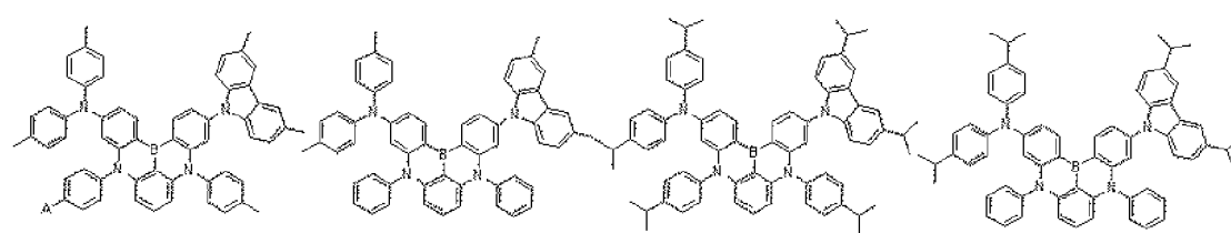
Dopant 77
