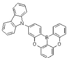
Dopant 185
