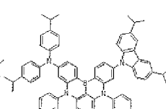
Dopant 80
