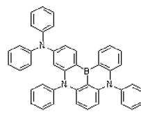
Dopant 51
