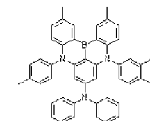
Dopant 83
