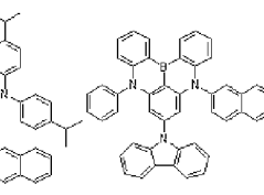
Dopant 96
