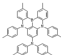
Dopant 47
