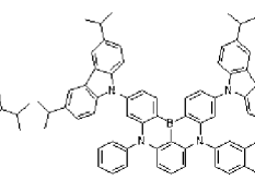
Dopant 110
