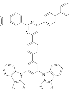
E11
