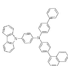
H5
