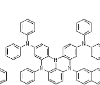
Dopant 91
