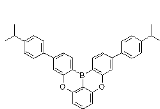
Dopant 177
