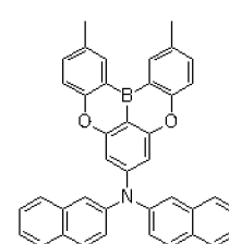
Dopant 216
