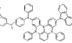
Dopant 76
