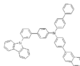
H16
