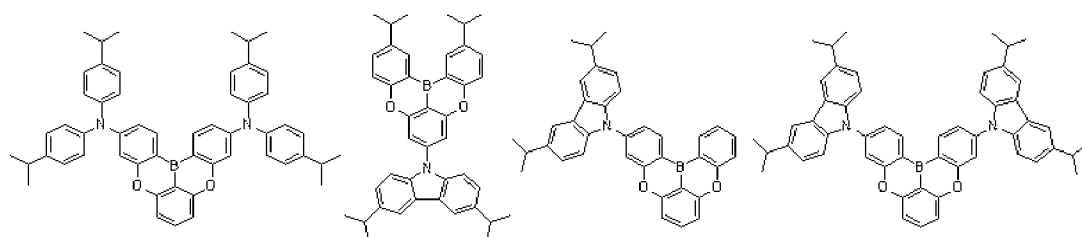
Dopant 197
