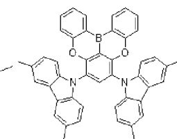
Dopant 228
