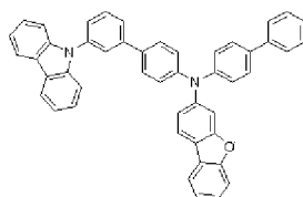
H18
