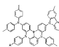
Dopant 77
