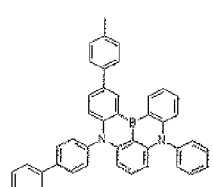
Dopant 38
