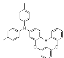
Dopant 189
