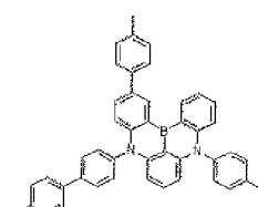
Dopant 37
