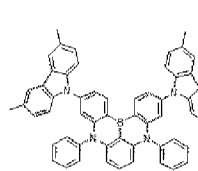
Dopant 73
