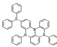
Dopant 51
