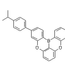
Dopant 179
