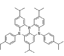
Dopant 138
