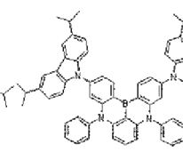
Dopant 75
