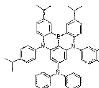
Dopant 85
