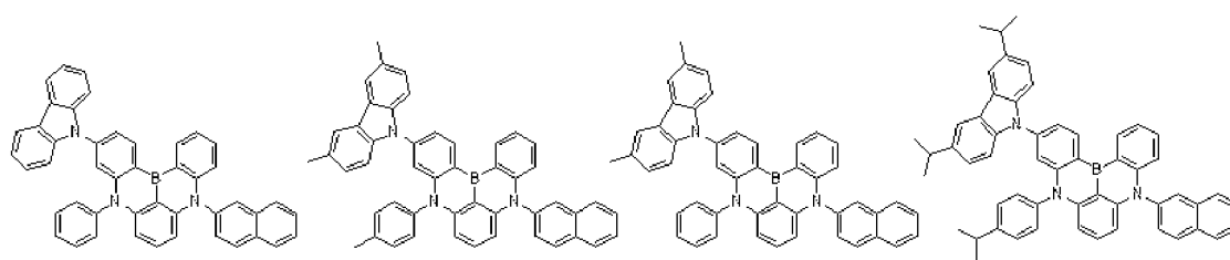
Dopant 101
