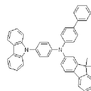
H11
