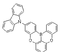
Dopant 185
