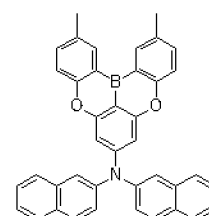
Dopant 216
