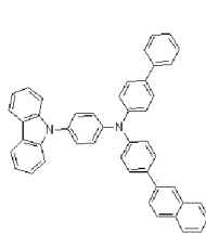
H2
