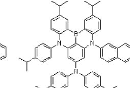
Dopant 84
