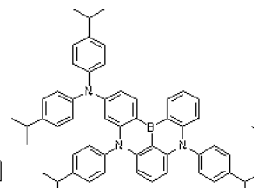
Dopant 54
