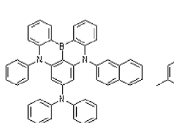
Dopant 81
