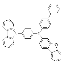
H14
