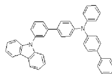
H7
