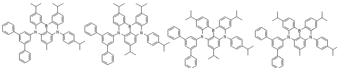
Dopant 149
