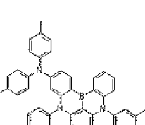
Dopant 87
