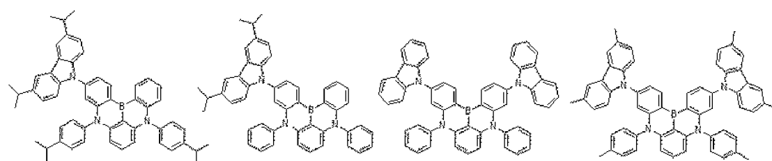
Dopant 69
