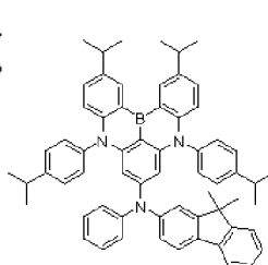
Dopant 120
