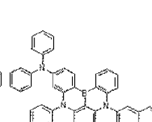
Dopant 86
