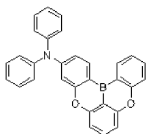
Dopant 182
