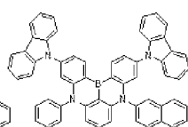
Dopant 106
