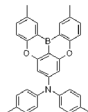
Dopant 188
