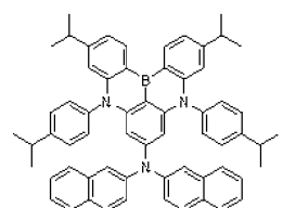
Dopant 141
