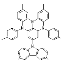
Dopant 62
