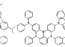
Dopant 111
