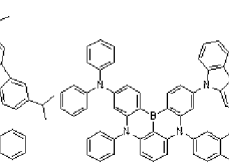
Dopant 111
