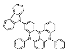
Dopant 66
