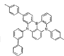
Dopant 32
