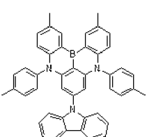
Dopant 63
