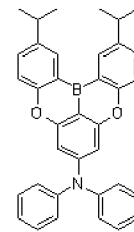
Dopant 204
