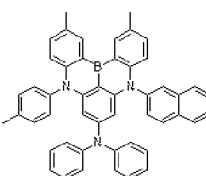
Dopant 83
