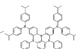
Dopant 60
