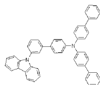
H17
