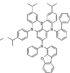
Dopant 118
