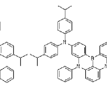
Dopant 95
