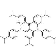
Dopant 139
