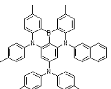
Dopant 82
