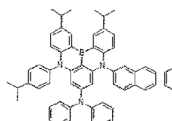
Dopant 85
