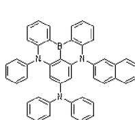
Dopant 81
