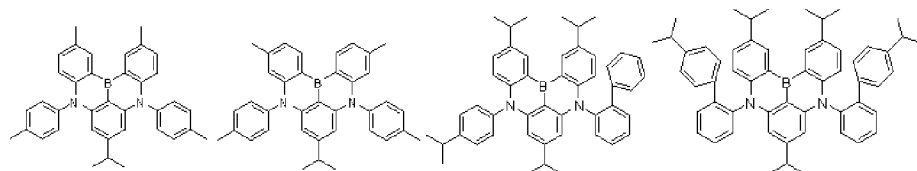
Dopant 145
