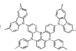
Dopant 72
