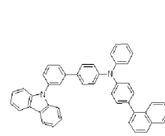
H4
