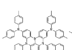
Dopant 93
