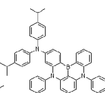
Dopant 55
