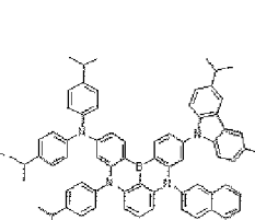
Dopant 114
