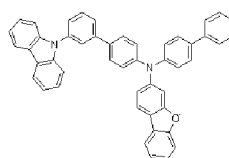
H18
