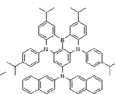
Dopant 140
