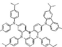
Dopant 79
