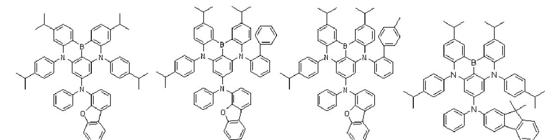
Dopant 117
