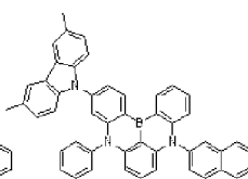
Dopant 103
