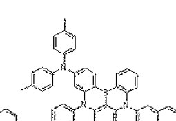
Dopant 88
