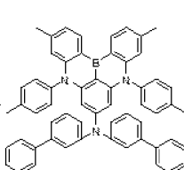
Dopant 143
