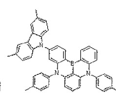
Dopant 67
