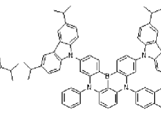
Dopant 110
