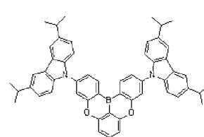
Dopant 200
