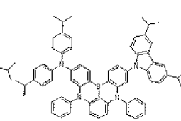
Dopant 80
