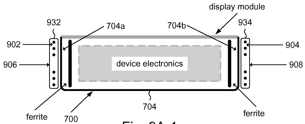
Fig. 9A-1
