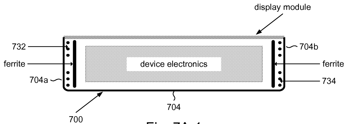
Fig. 7A-1
