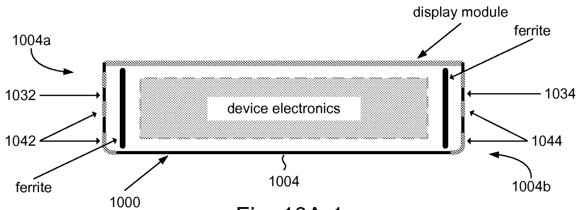
Fig. 10A-1
