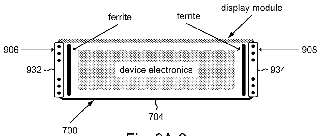
Fig. 9A-2
