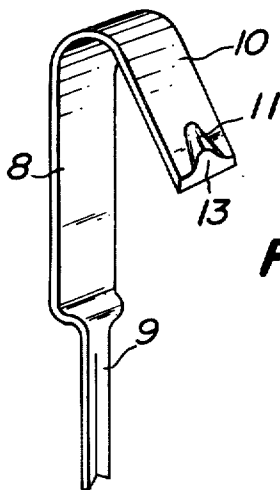
FIG. 2a
