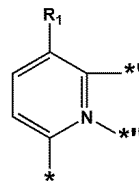
<화학식 2-1(3)>
