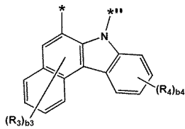
<화학식 2-8>
