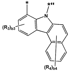
<화학식 2-8>
