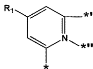
<화학식 2-1(2)>
