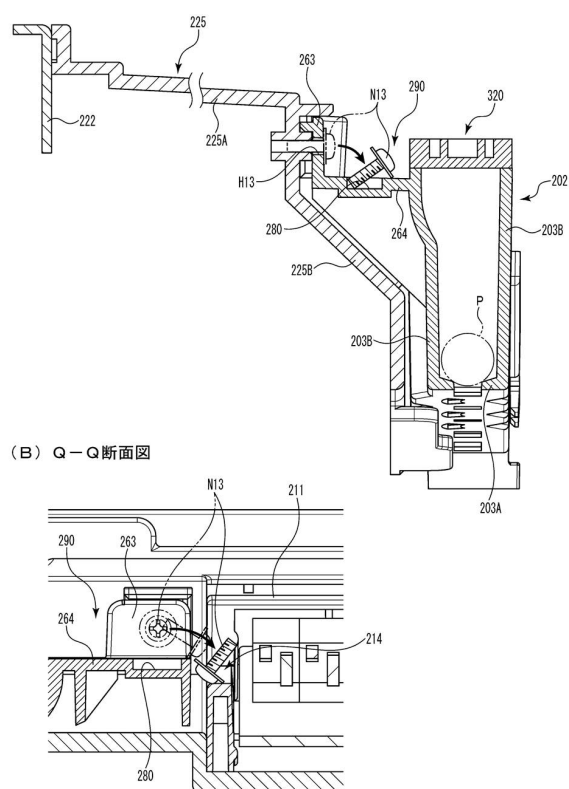
(A) P-P断面図
