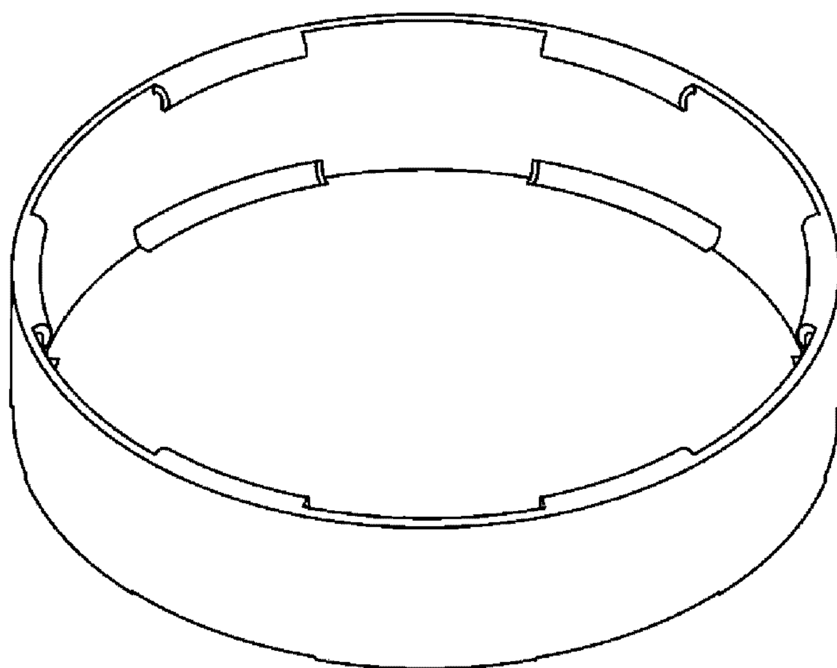
【立體圖】
