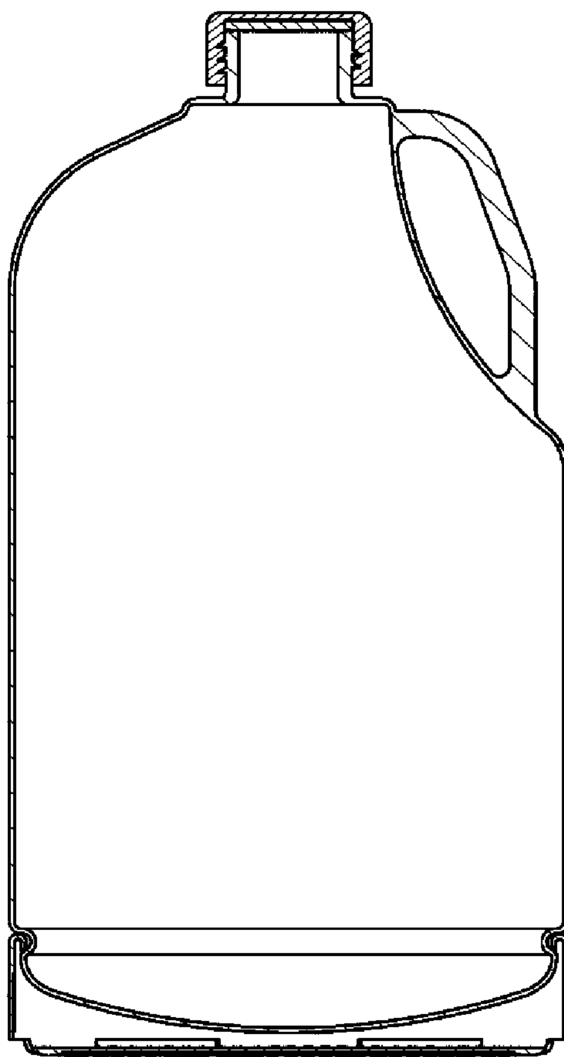
【B-B' 剖面參考圖】
