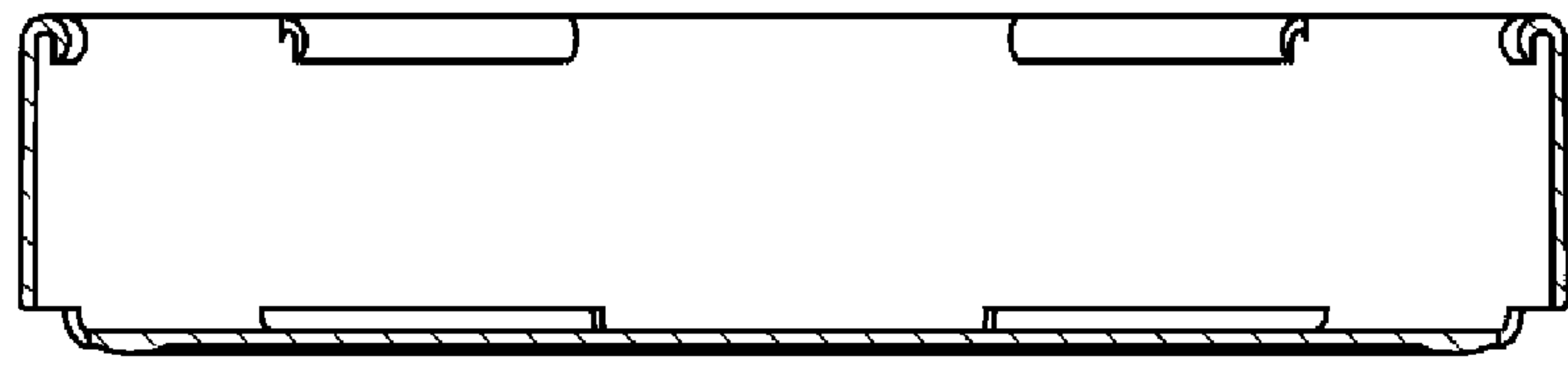
【A-A’ 剖面圖】
