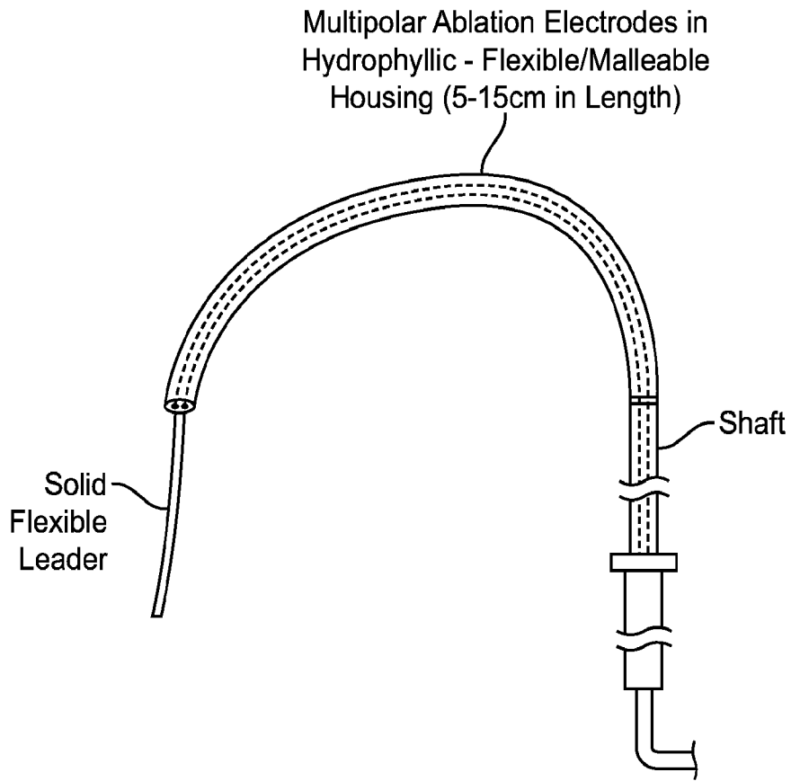
FIG. 9B
