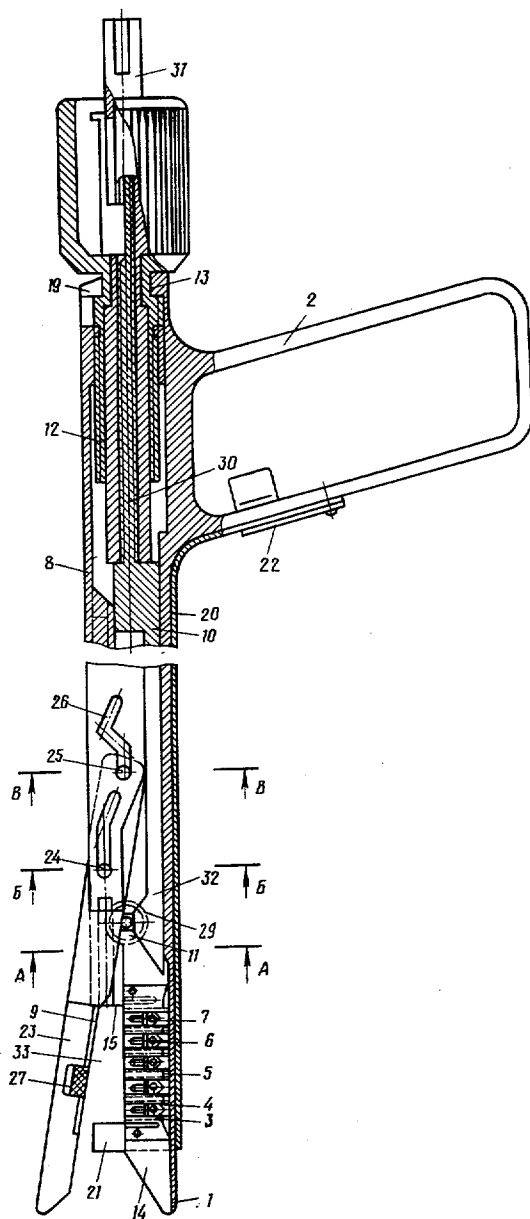
Фиг. 1
