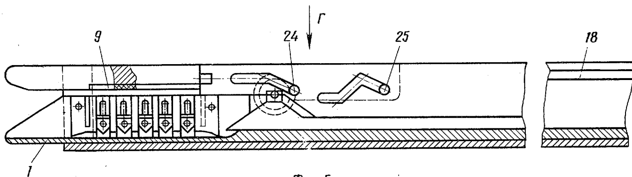
Фиг. 5
