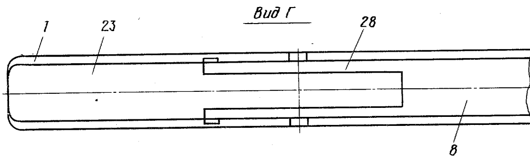
Фиг. 6
