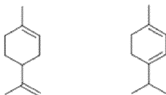
Limonene
