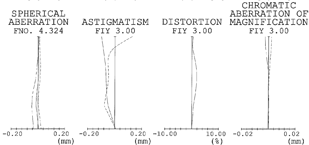
FIG.15I FIG.15J FIG.15K FIG.15L
