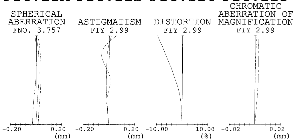
FIG. 22E FIG. 22F FIG. 22G FIG. 22H
