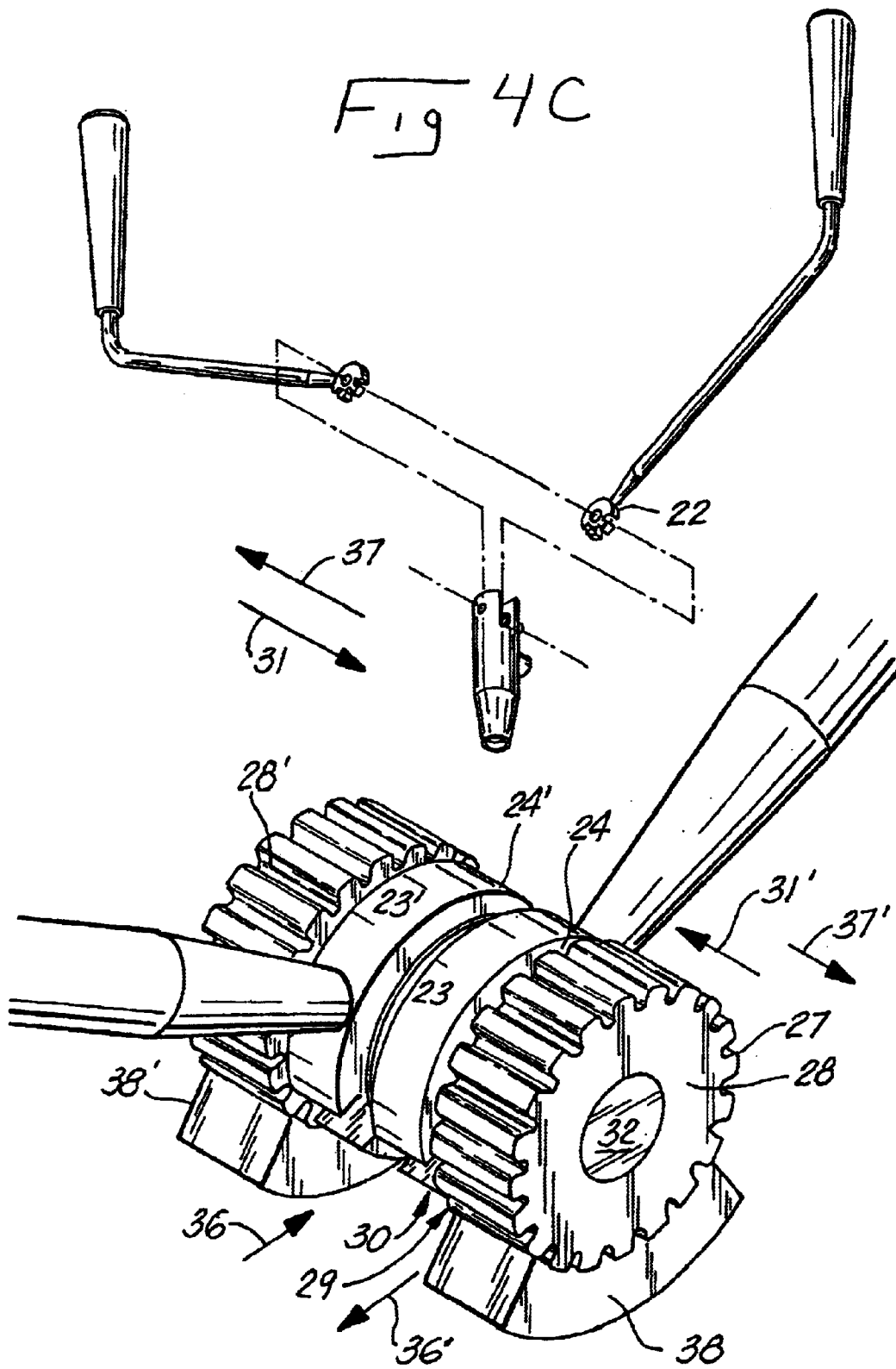
FIG. 4 D
