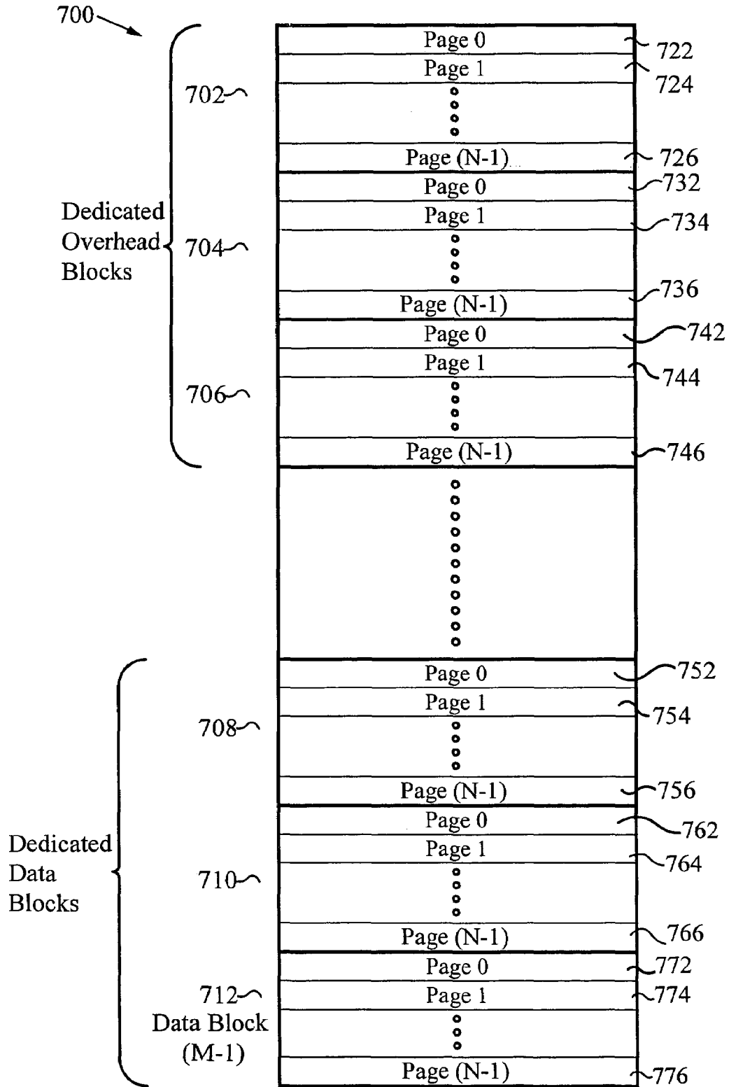
Flash Memory Array Fig. 7
