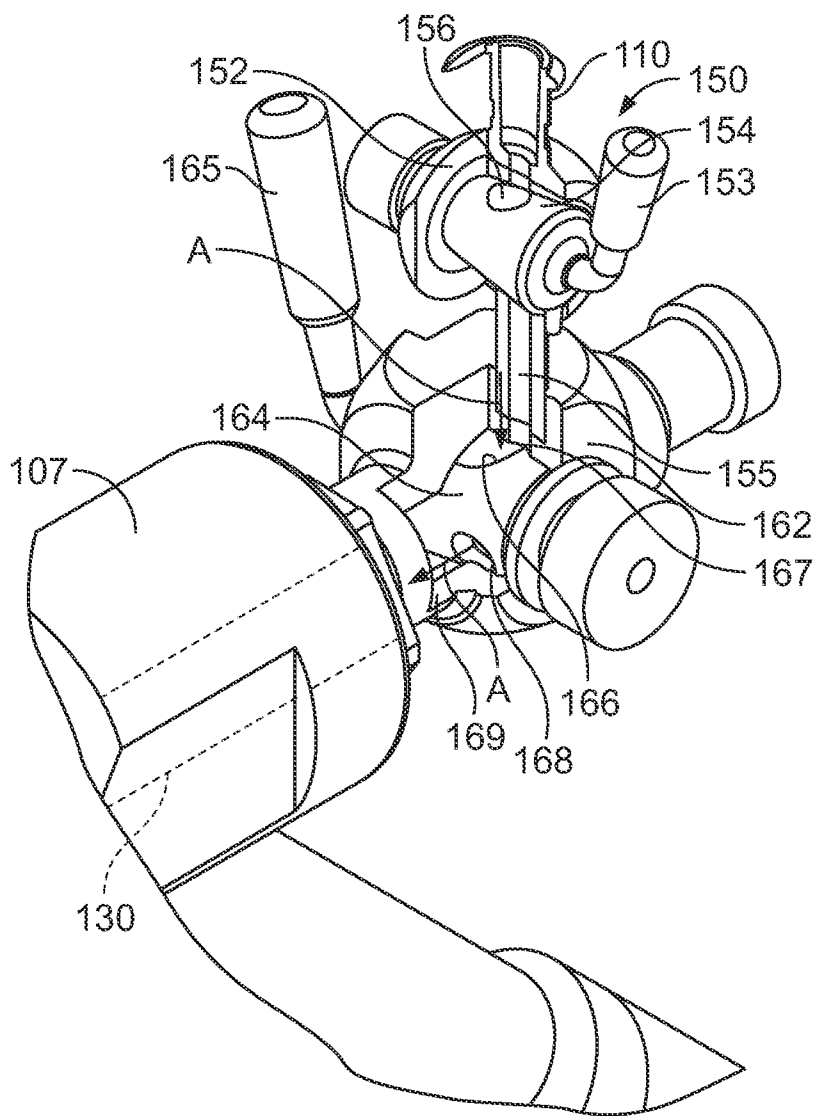
FIG. 6A
