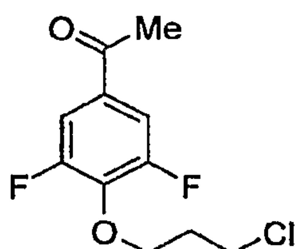
1-[4-(3-Chloropropoxy)-3,5-difluorophenyl]-ethanone
