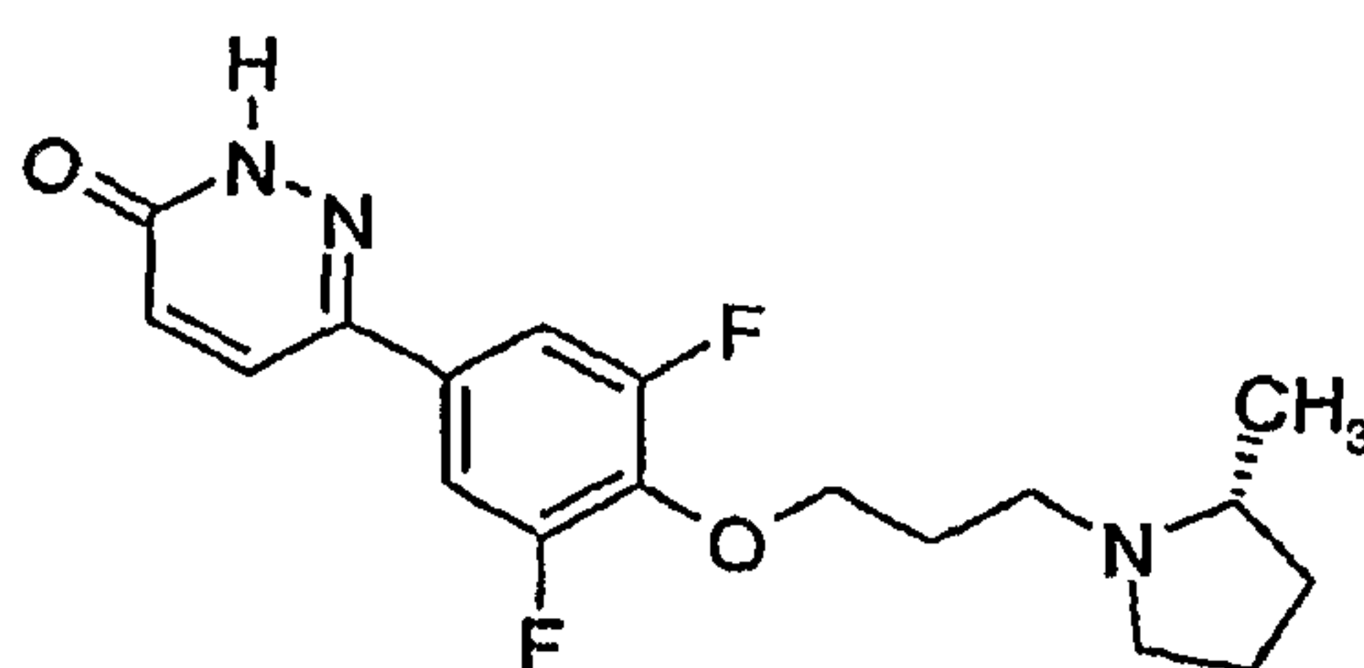
6-[3,5-Difluoro-4-[3-((R)-2-methylpyrrolidin-1-yl)-propoxy]-phenyl]-2H-pyridazin-3-one
