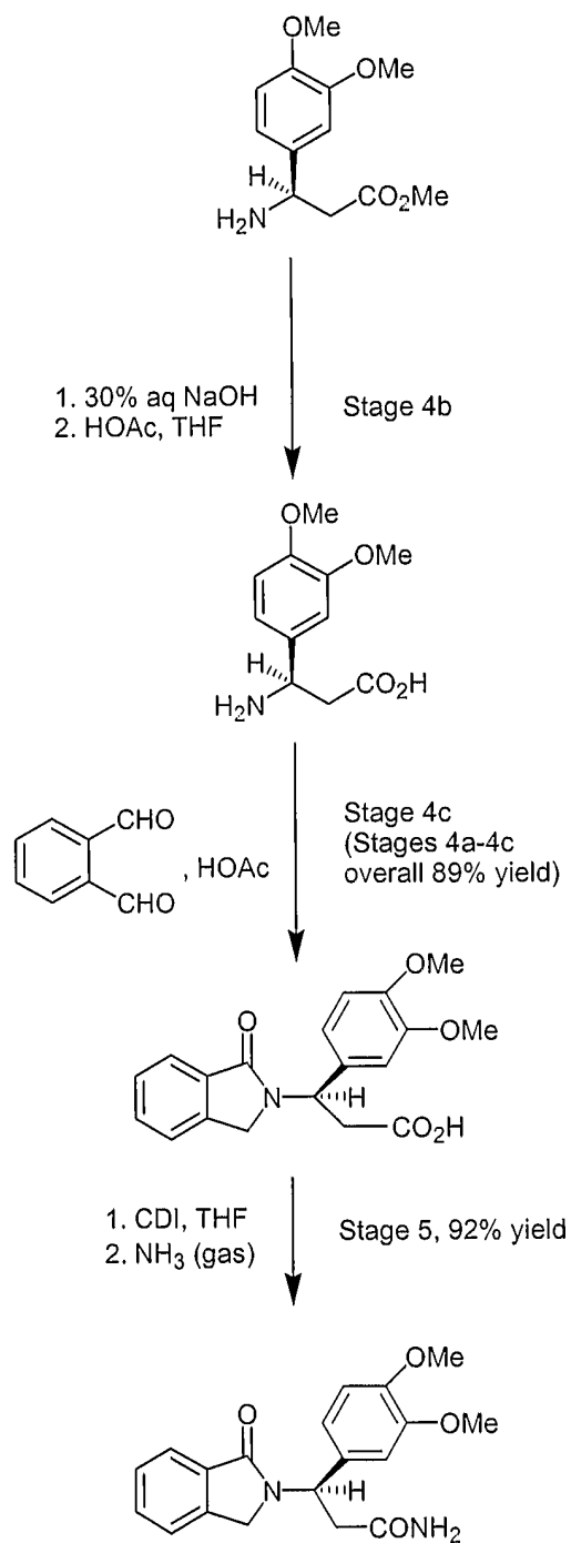
(-)-3-(3,4-dimethoxy-phenyl)-3-(1-oxo-1,3-dihydro-isoindol-2-yl)-propionamide
