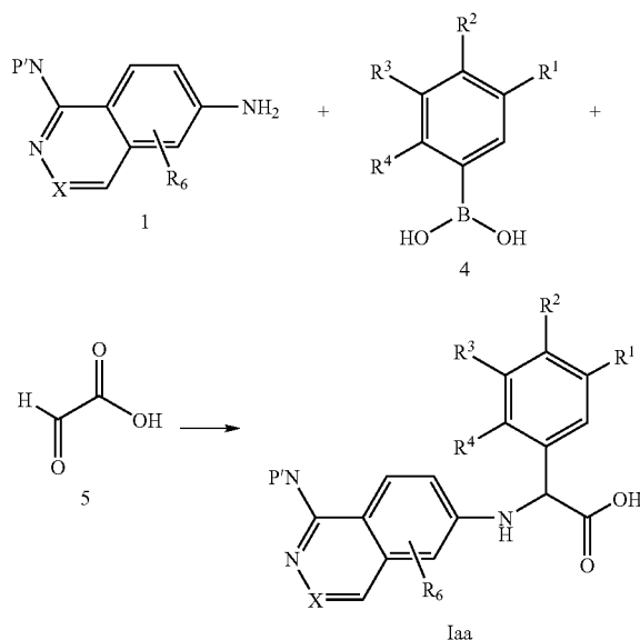
Scheme 2a
