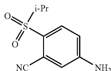
290A: 5-Amino-2-(isopropylsulfonyl)benzonitrile
