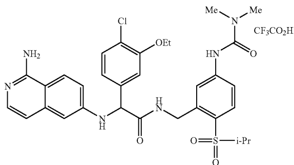
290A: 5-Amino-2-(isopropylsulfonyl)benzonitrile
