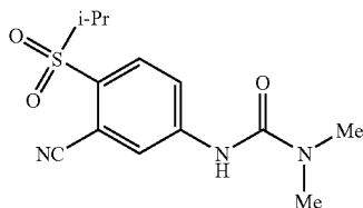
290B: 3-(3-Cyano-4-(isopropylsulfonyl)phenyl)-1,1-dimethylurea
