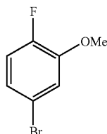
69A: 4-Bromo-2-methoxy-1-fluorobenzene
