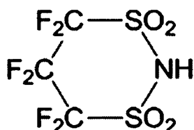
Structural Formula (D)
