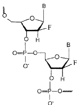
2'-F
