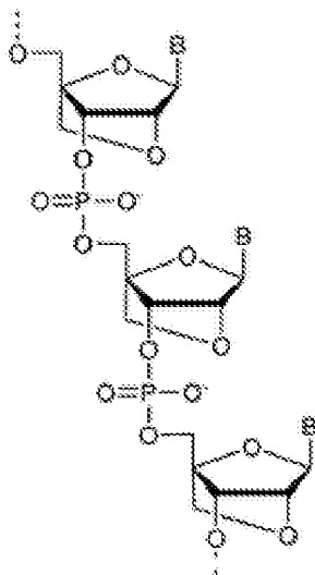
LNA
