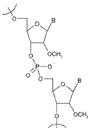
2' O-Me
