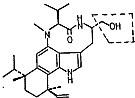
Teleocidin B 4
