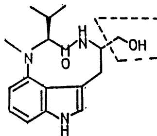
Indolactam V
