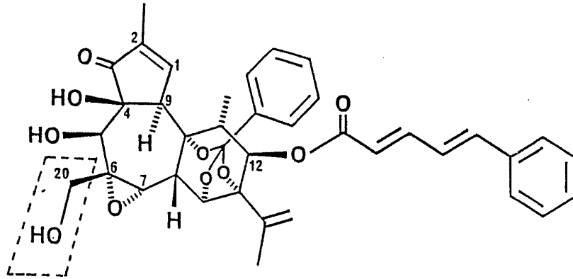
MEZEREIN
