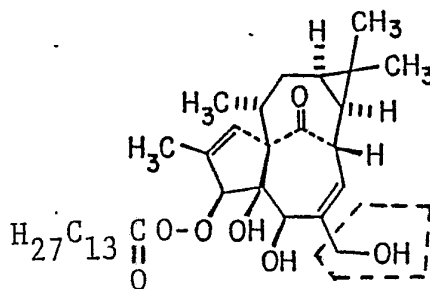
Ingenol 3-Tetradecanoate
