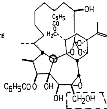
Gnidimacrin
