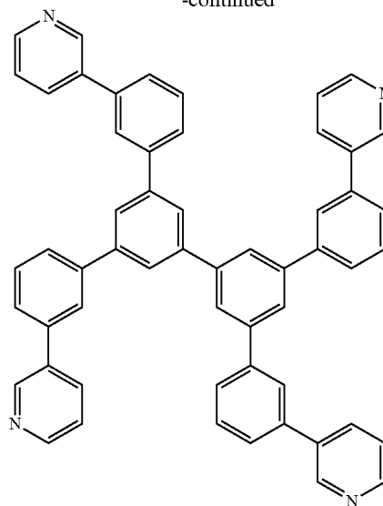
BP4mPy
