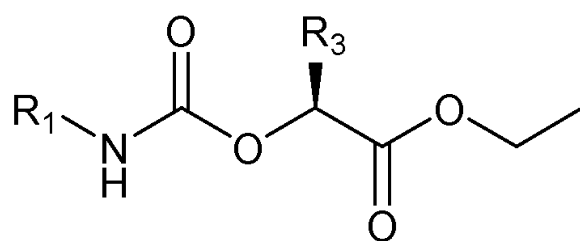
(Va);
