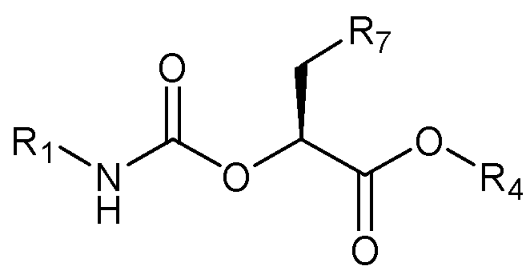
(IIIa);
