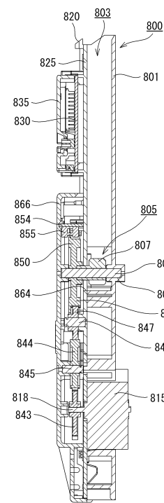
A-A断面図
