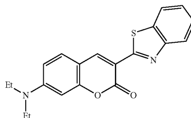
Coumarin 6
