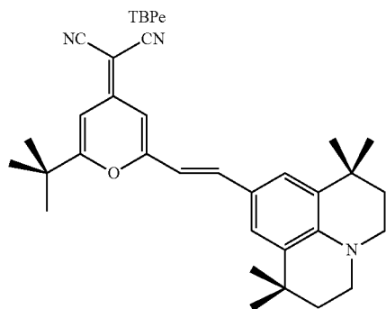
DCJTB
