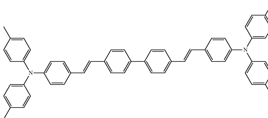
DPAVBi
