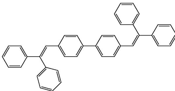
DPVBi
