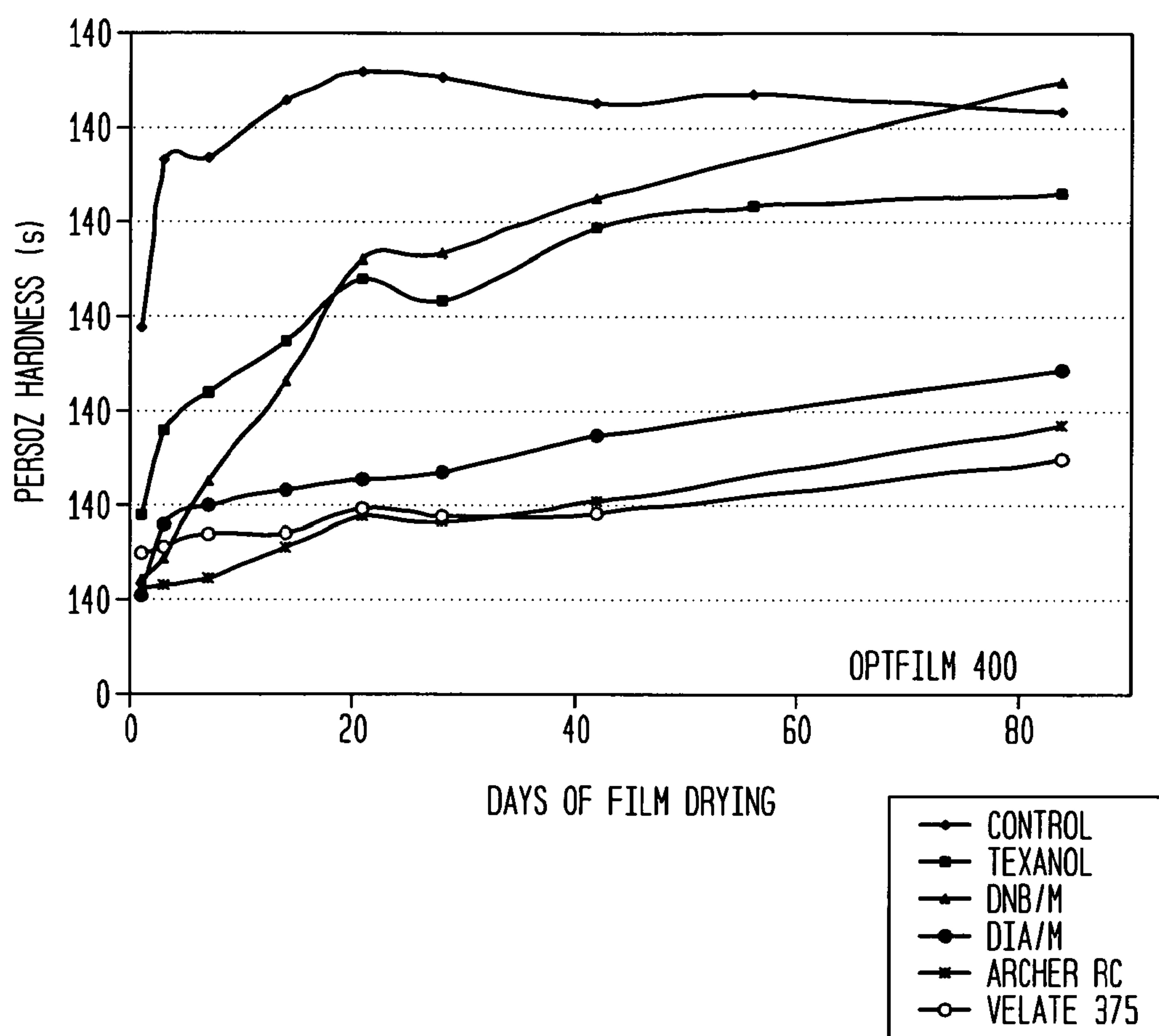
FIG. 12 PERSOZ HARDNESS
