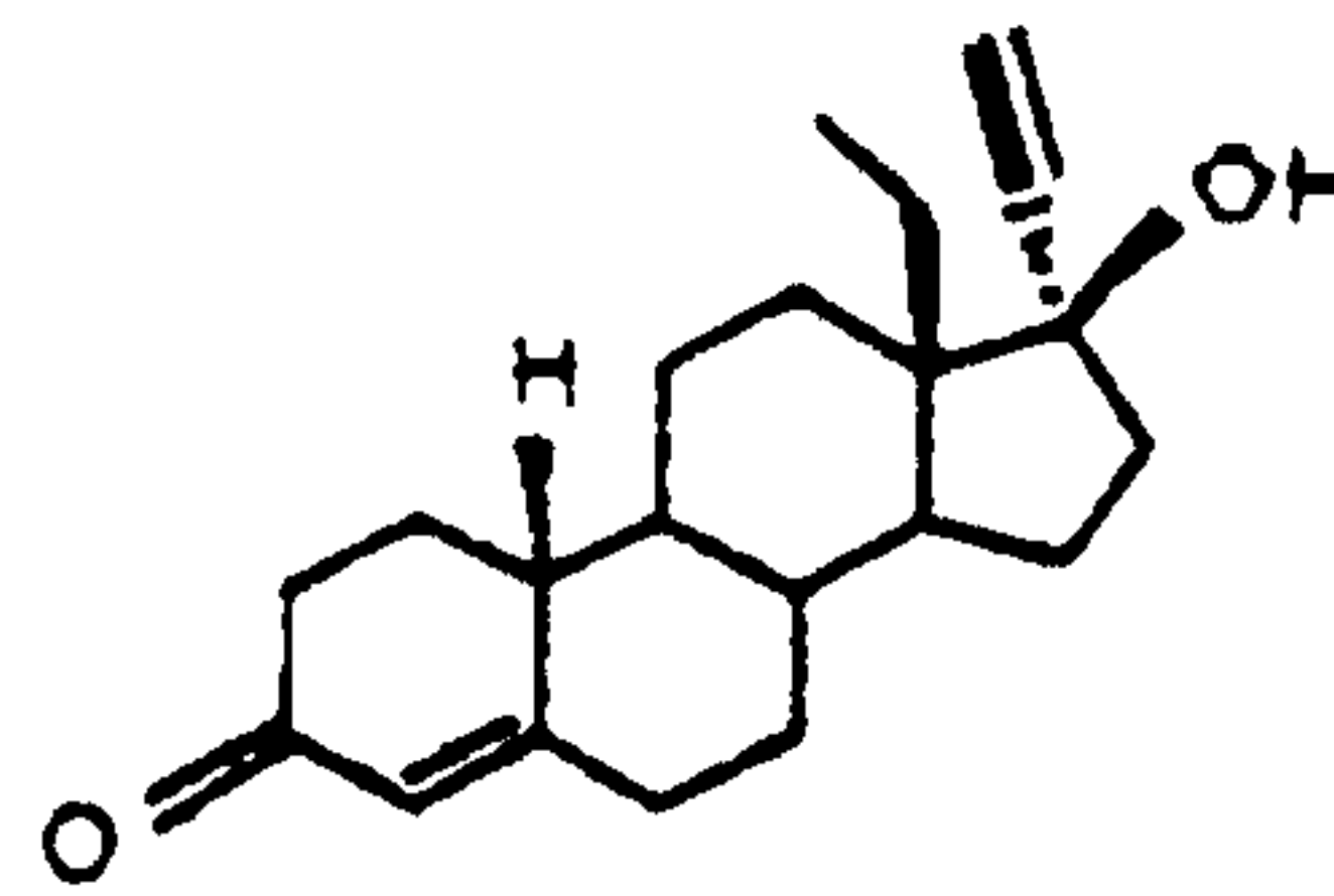
NORGESTREL
