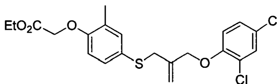
9-A
