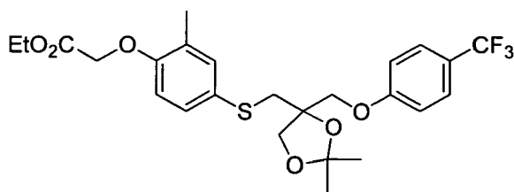
32-B
