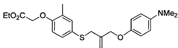
12-A
