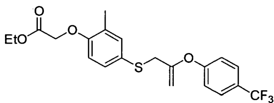
23-C
