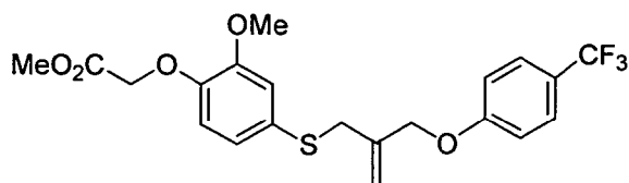
16-A
