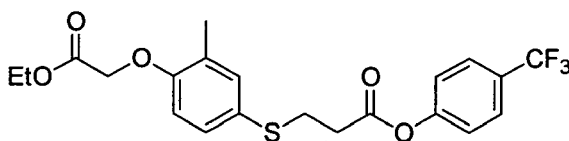
22-B
