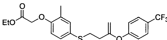
22-C
