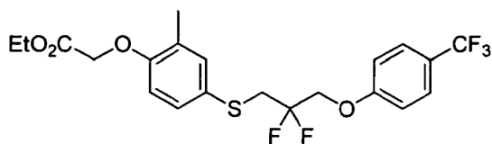
30-A
