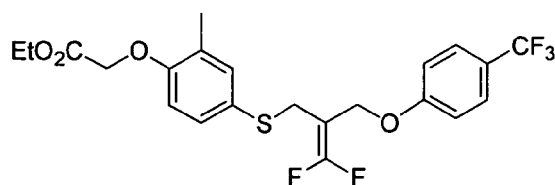
18-D
