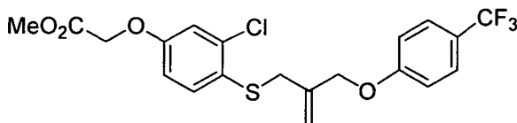
15-C
