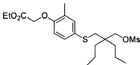
29-D
