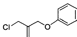
5-B (2-Chloromethyl-allyloxy)-benzene
