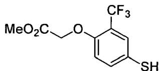
14-B
