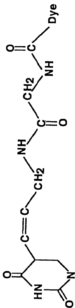
Diglycinyllinker
