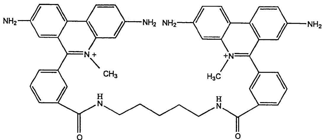
meta -EthD
