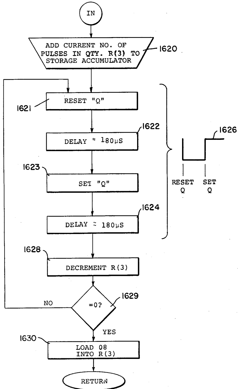
Fig. 53. OUTPUT 16 Hz
