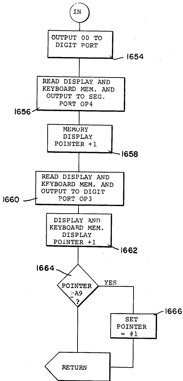
Fig. 56. MUX DISPLAY
