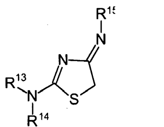
(Ca-IV)
