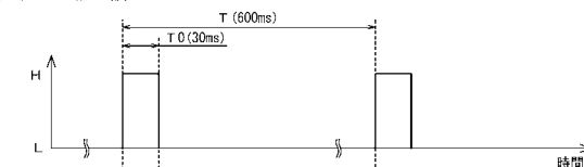
(a) TC点の論理
