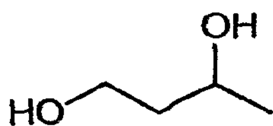
1,3-Butanediol
