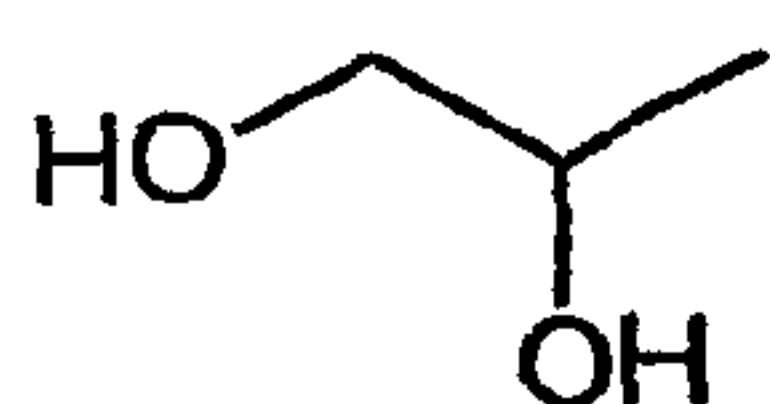
1,2-Propanediol
