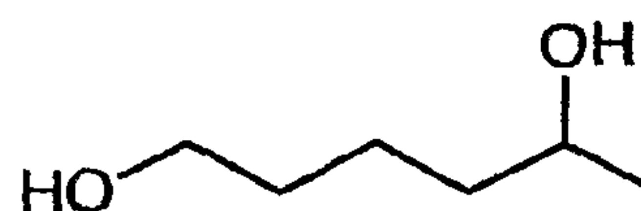
1,5-Hexanediol
