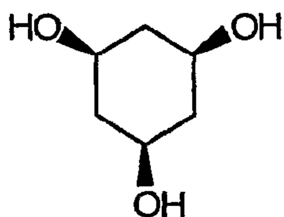
cis-1,3,5-Cyclohexanetriol
