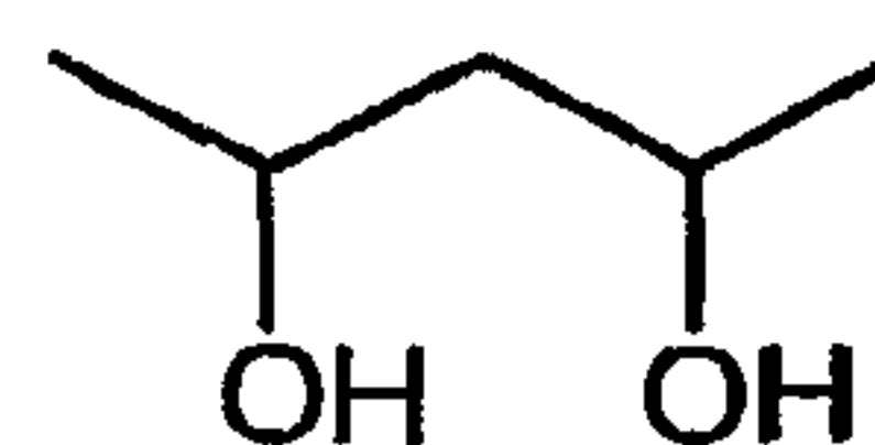
2,4-Pentanediol
