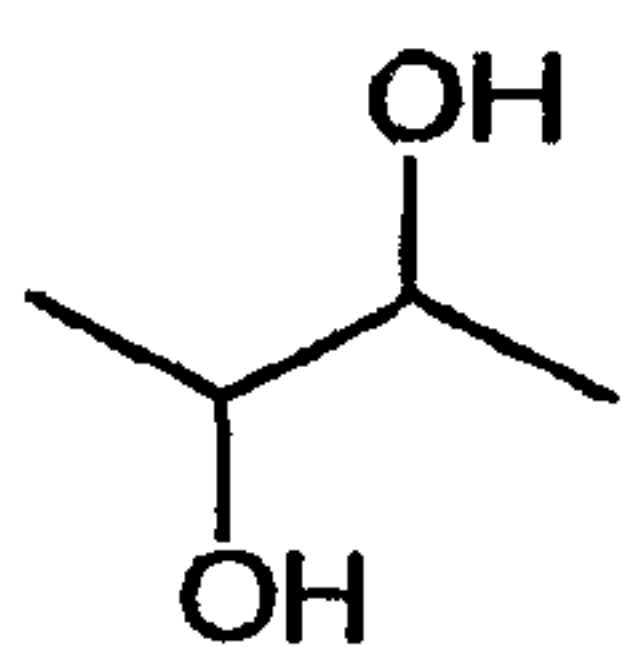
2,3-Butanediol
