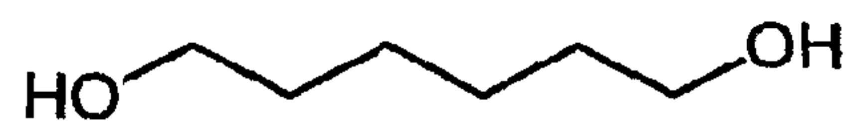
1,6-Hexanediol
