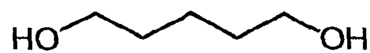
1,5-Pentanediol
