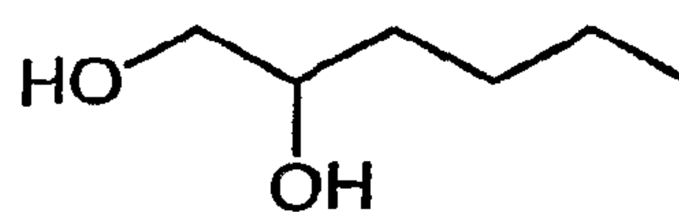
1,2-Hexanediol
