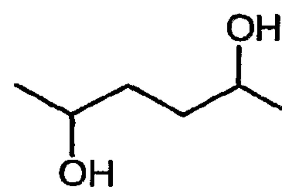
2,5-Hexanediol
