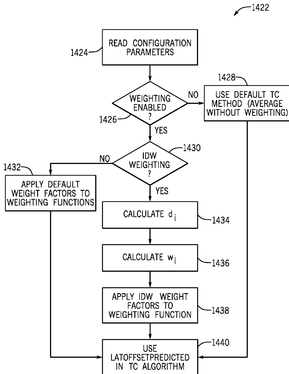
FIG. 14C
