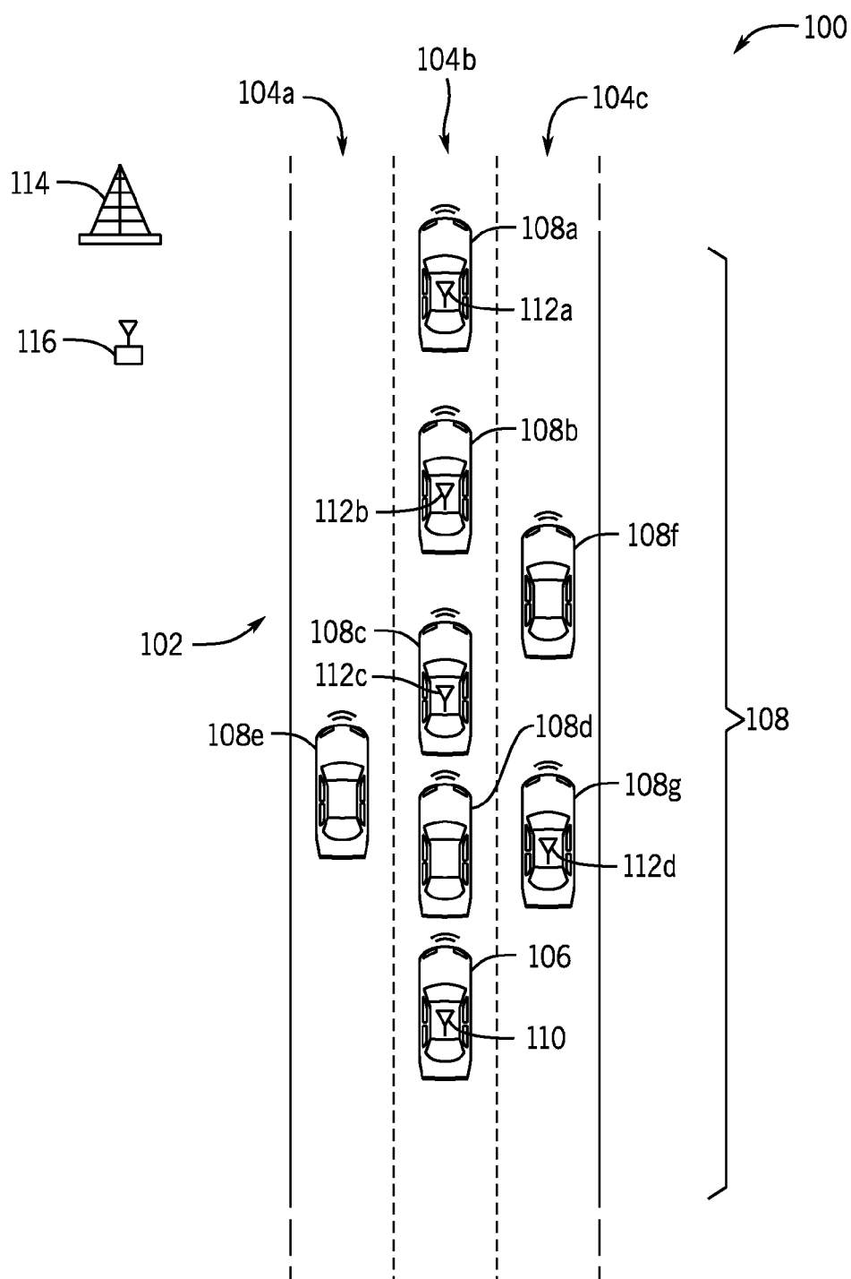
FIG. 1A
