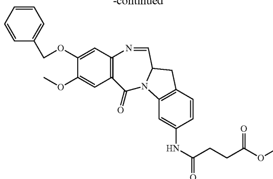
266a
