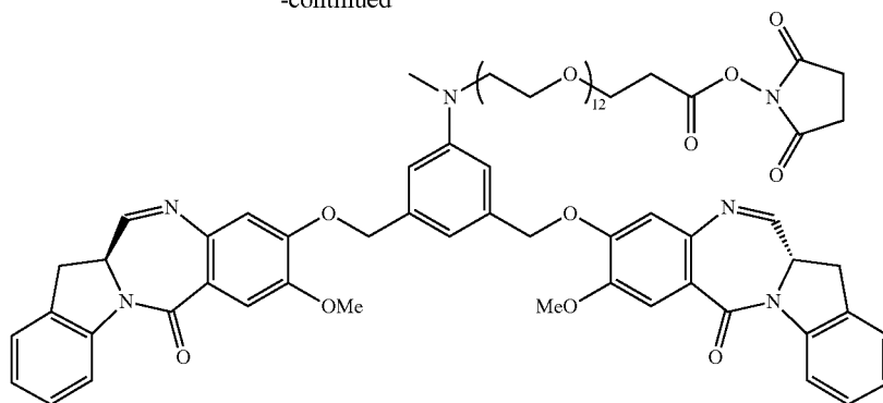
265g
