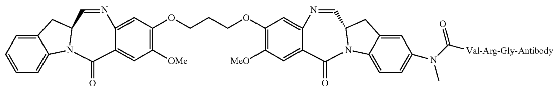
Dimer 6
