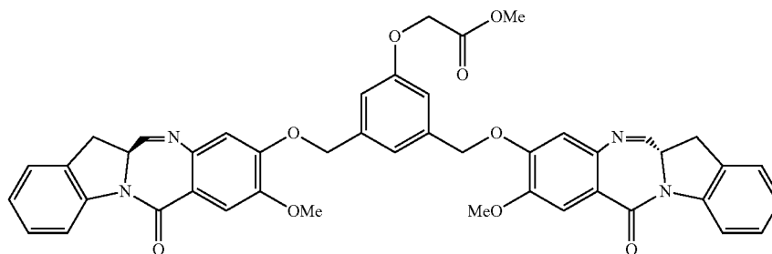
36 (IGN-05)
