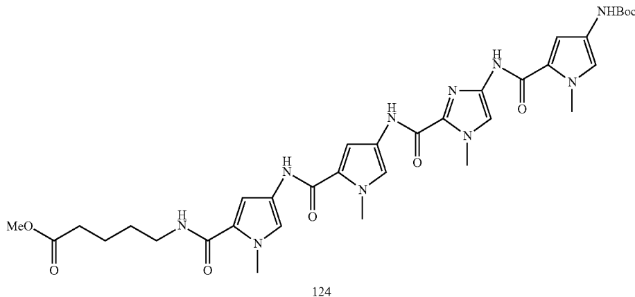
124
