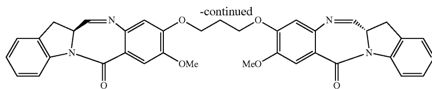
15 (IGN-09)
