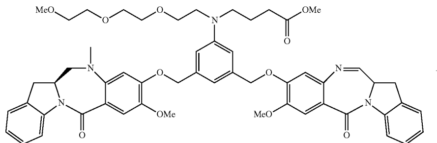
256d (IGN-29-OMe)
