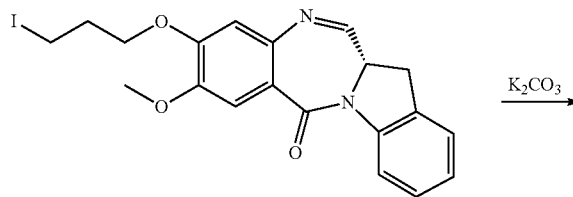
258g
