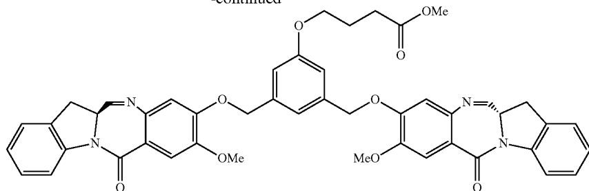
35 (IGN-04)
