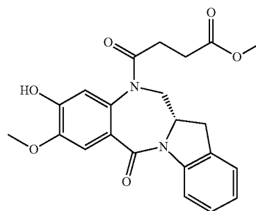
260b
