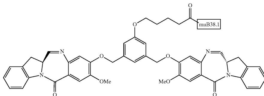
B38.1-IGN-03
