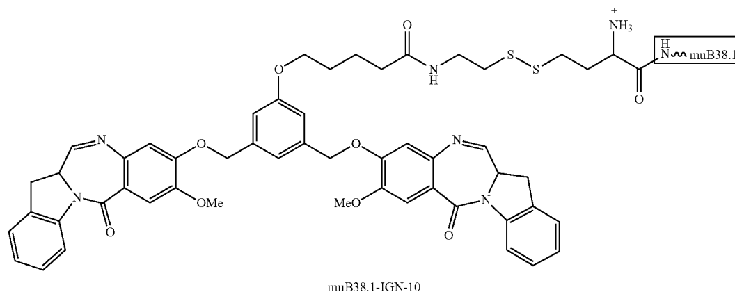
muB38.1-IGN-10
