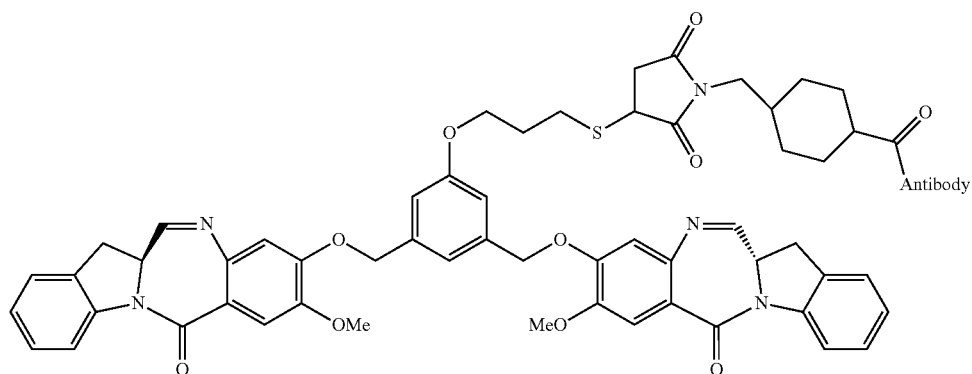
Dimer 3
