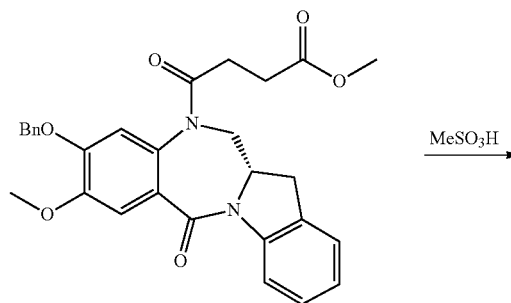
260a
