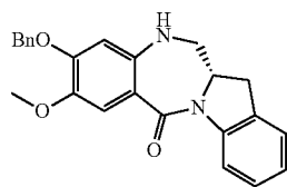
256a
