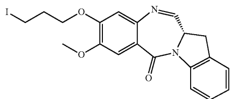
258g
