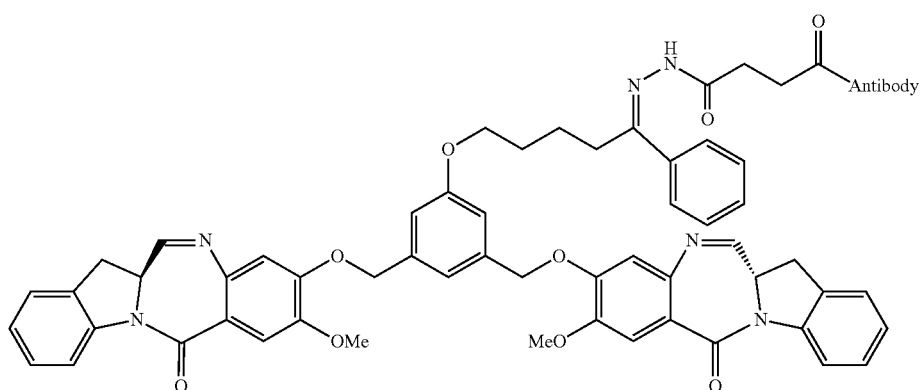
Dimer 4
