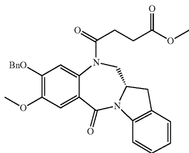
260a
