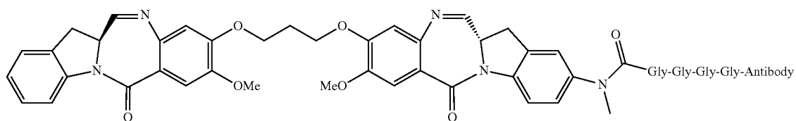
Dimer 5
