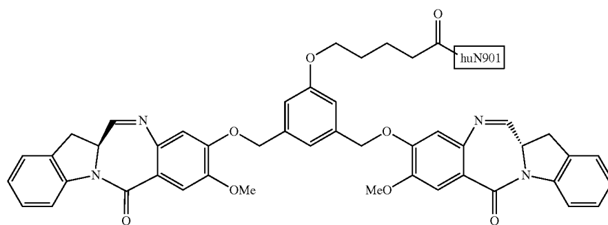
N901-IGN-03
