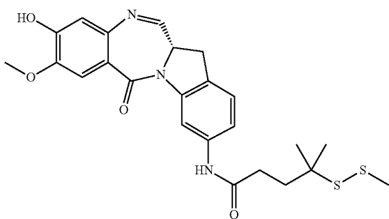
258f
