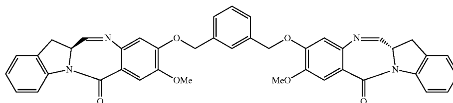
18 (IGN-01)
