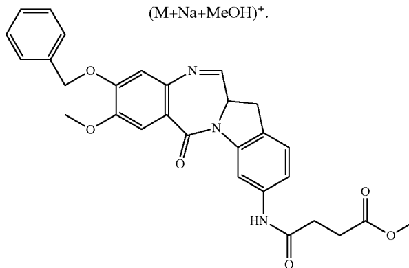
266a
