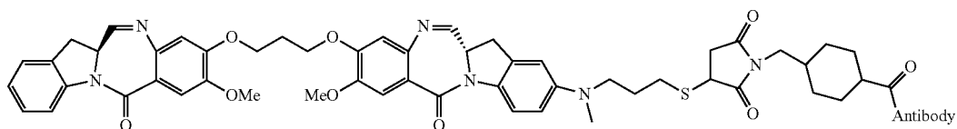
Dimer 7
