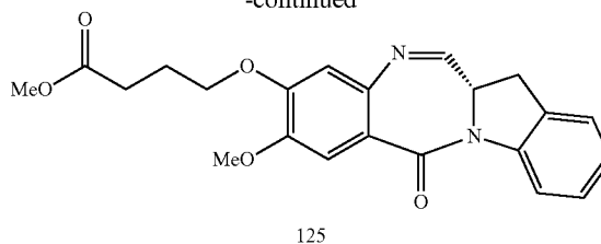
125
