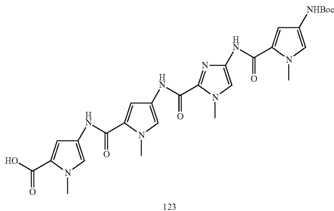
123
