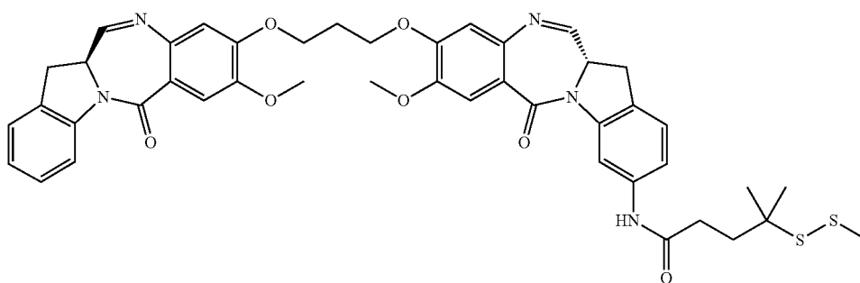
258h
