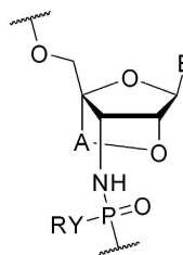
(V')
