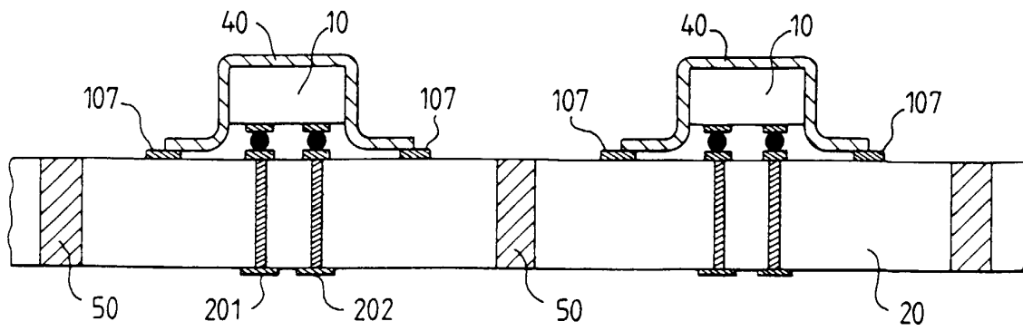
COUPE AA' FIG. 3b
