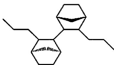
MESO BODY
