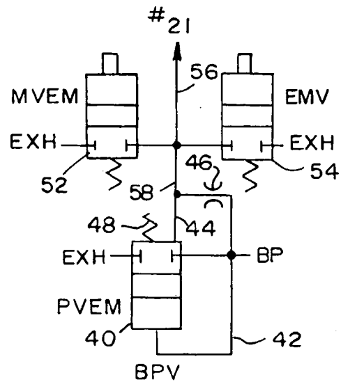
FIG. 5 (Técnica anterior)
