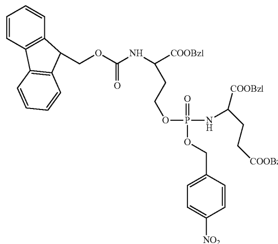
2 MW955.94
