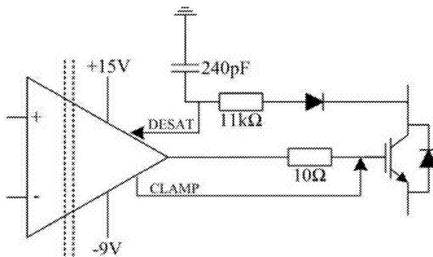
Infiniteon 1ED020112-F
