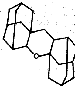
Trans-type
