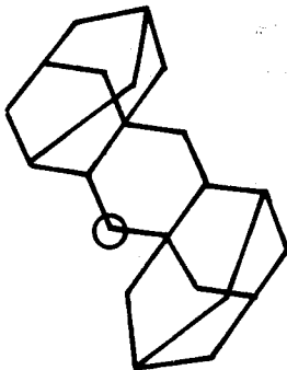
Trans-type
