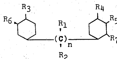
di(cyclohexyl)alkane
