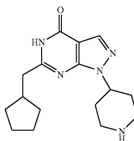
Example 195
