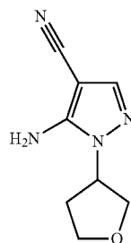
Enantiomer B
