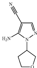
Enantiomer A
