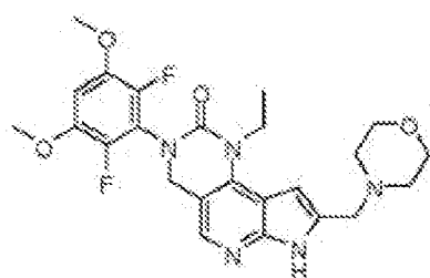
Forbindelse 1.
