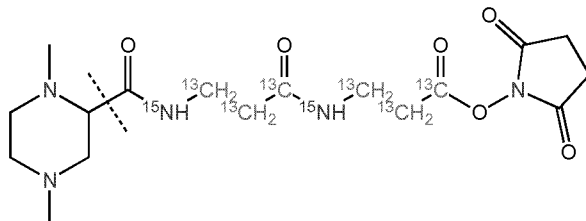
TMT-1-21-114.10436 (Subset 2)
