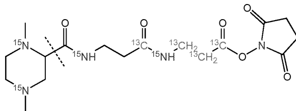
TMT-1-21-115.10771 (Subset 3)
