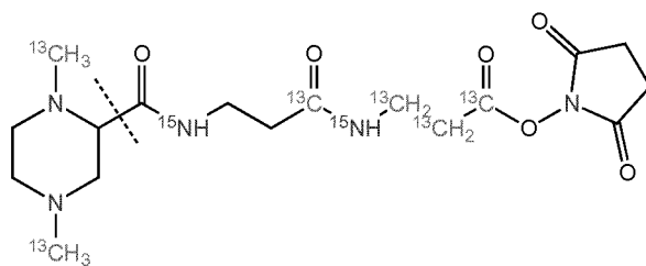
TMT-1-21-116.10475 (Subset 4)
