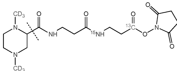
TMT-4-3-120.14834 (Subset 8)
