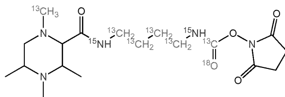
TMT-6-27-143.13269 (Subset 3)
