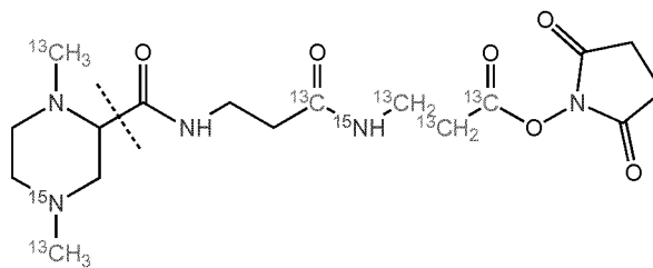
TMT-1-21-116.11107 (Subset 4)
