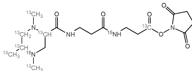
CN(C)C(=O)NCCC(=O)NCC(=O)OC1C(=O)N2C(=O)CCC2N1C
