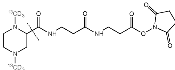
TMT-4-3-121.15169 (Subset 9)
