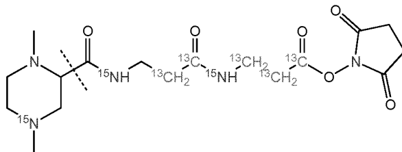
TMT-1-21-114.10436 (Subset 2)
