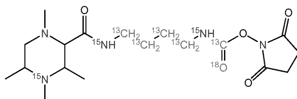
TMT-6-27-142.14198 (Subset 2)
