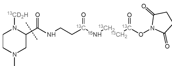
TMT-2-7-1-117.12659 (Subset 5)
