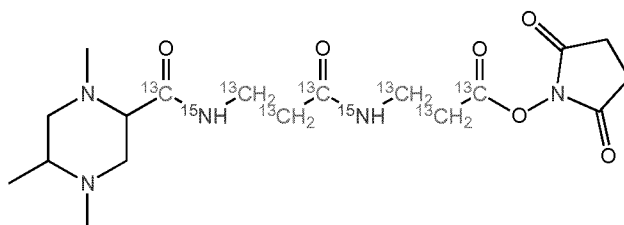
TMT-5-24-128.12001 (Subset 2)
