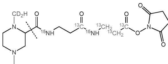
TMT-2-7-115.11988 (Subset 3)
