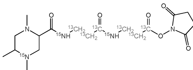
TMT-5-24-128.12633 (Subset 2)
