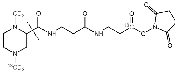
TMT-4-3-121.15169 (Subset 9)
