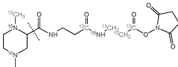
TMT-1-21-116.11107 (Subset 4)
