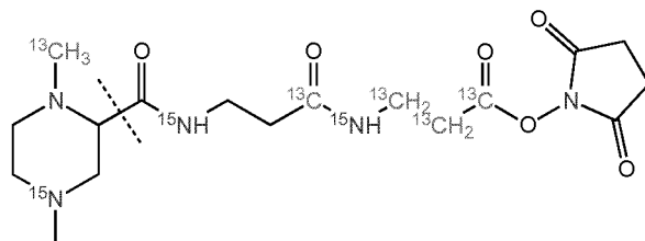
TMT-1-21-115.11403 (Subset 3)
