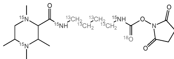
TMT-6-27-143.13901 (Subset 3)
