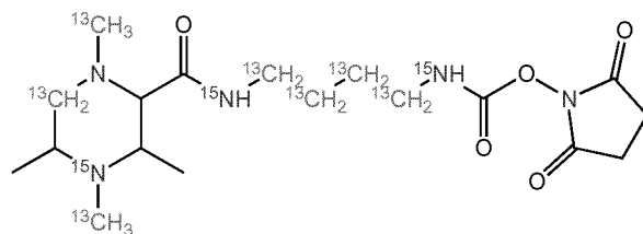
TMT-6-27-145.15204 (Subset 5)
