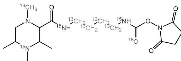
TMT-6-27-143.14533 (Subset 3)
