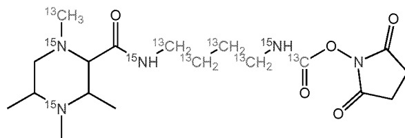
TMT-6-27-144.13605 (Subset 4)
