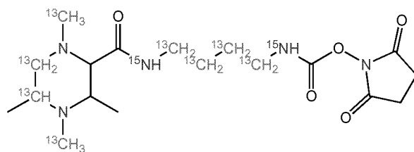
TMT-6-27-146.14276 (Subset 6)
