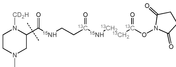
TMT-2-7-1-116.12323 (Subset 4)
