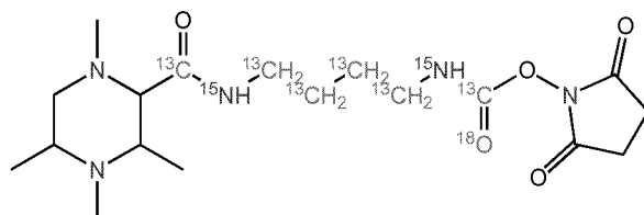
TMT-6-27-142.13566 (Subset 2)
