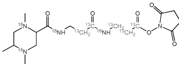
TMT-5-24-129.11704 (Subset 3)
