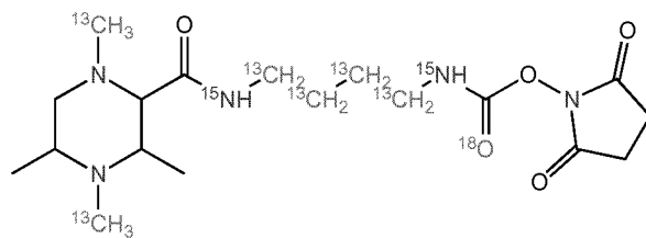
TMT-6-27-144.13605 (Subset 4)
