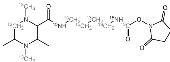
TMT-6-27-145.1394 (Subset 5)
