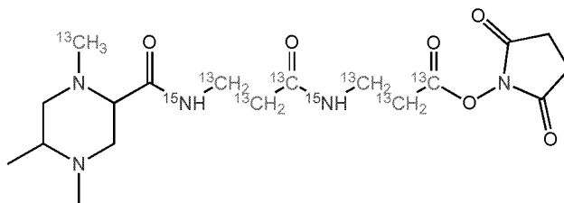
TMT-5-24-129.11704 (Subset 3)
