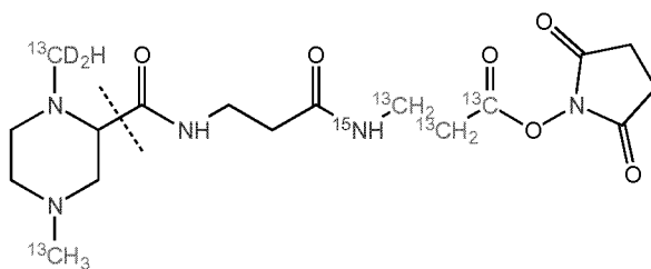
TMT-2-7-1-118.12994 (Subset 6)
