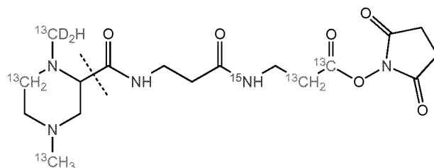
TMT-2-7-119.1333 (Subset 7)
