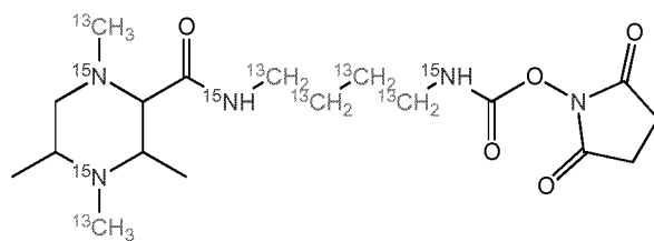
TMT-6-27-145.14572 (Subset 5)
