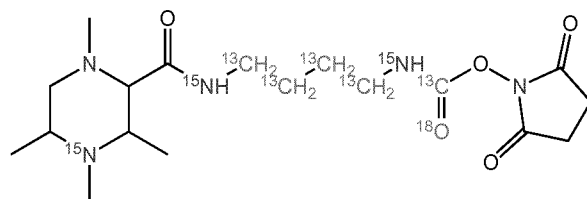
TMT-6-27-142.14198 (Subset 2)
