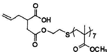
Macromonomer E5
