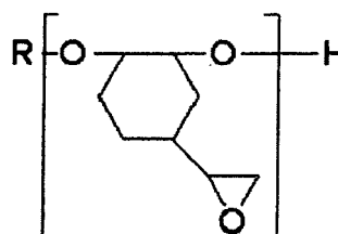
EHPE-3150
