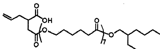
Macromonomer A5
