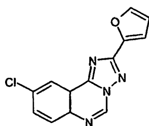
CGS-15943
