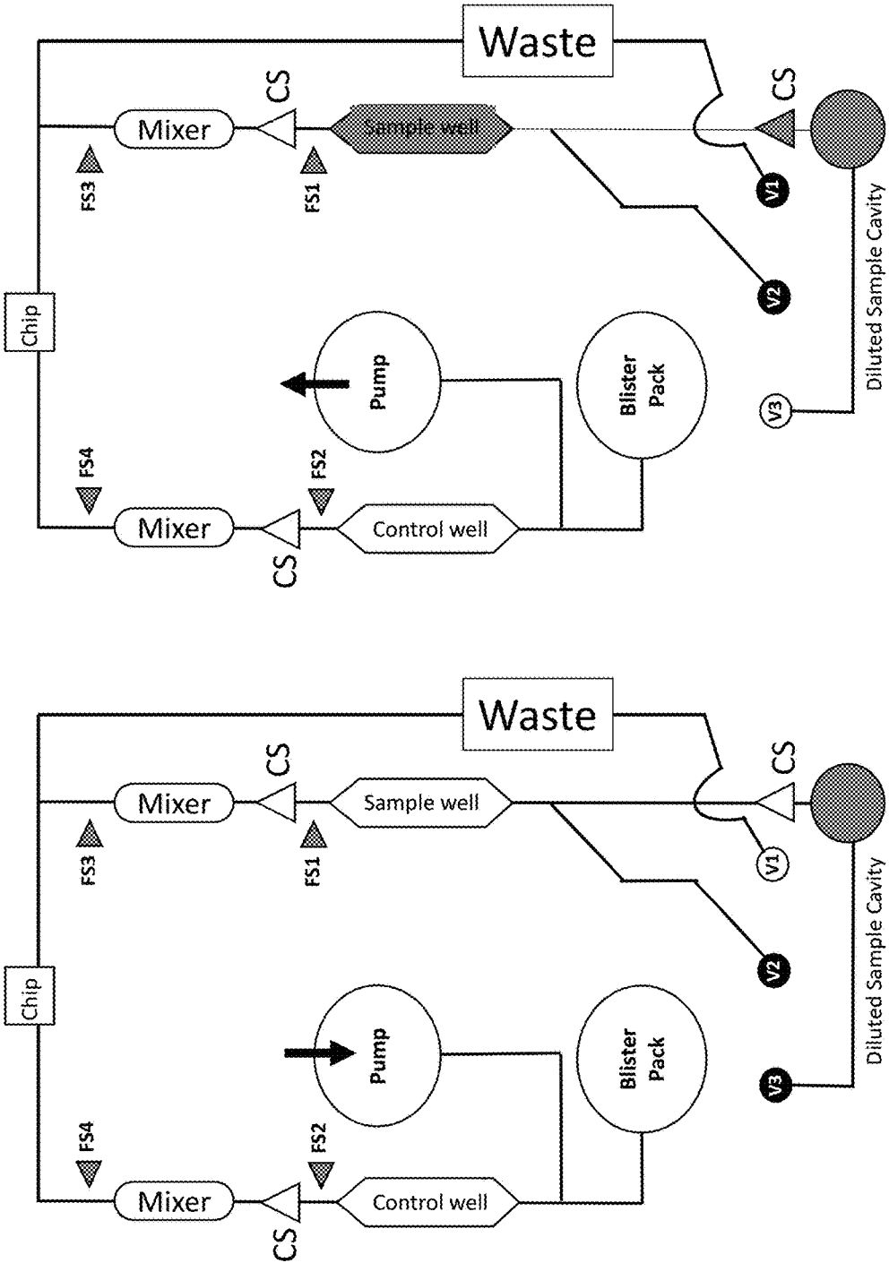
FIG. 20C (Prime pump)
