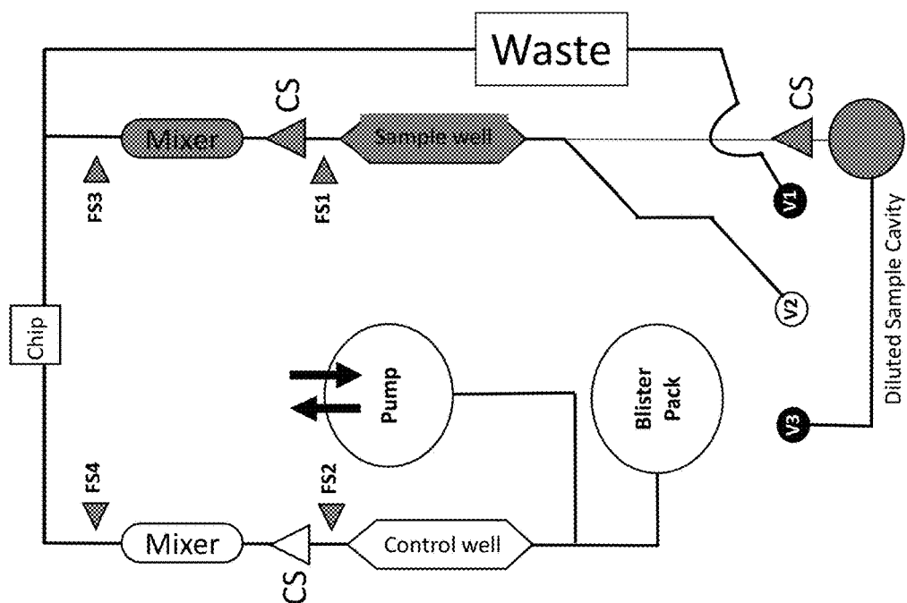
FIG. 20F (Mix)
