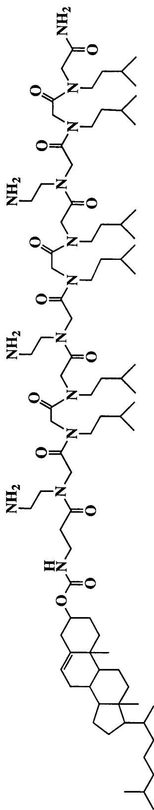
Chol-β-ala-(NaeNiaNia) 3
