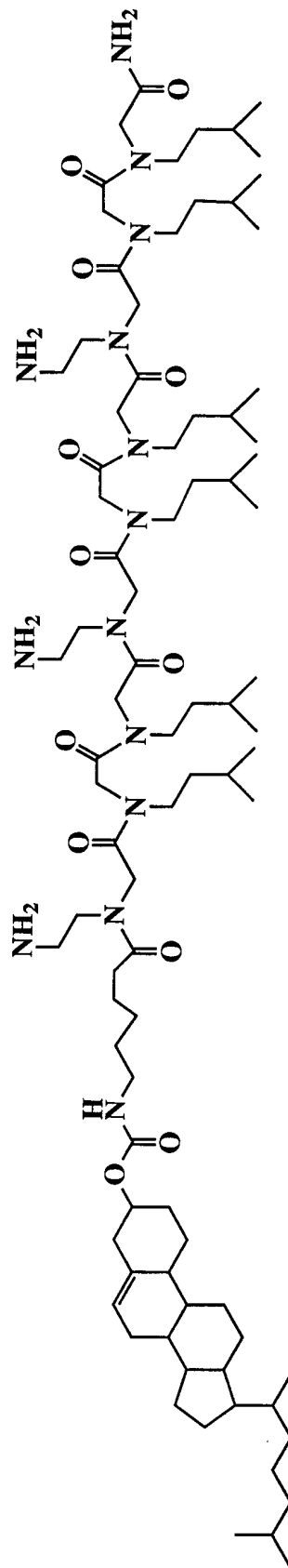
Chol-Ahx-(NaeNiaNia) 3
