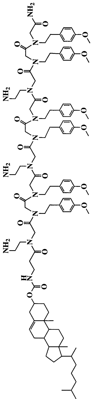
Chol-β-ala-(NaeNmpeNmpe) 3
