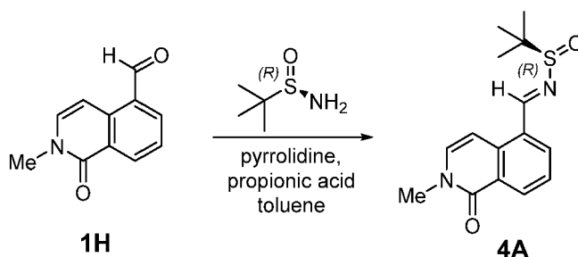
Scheme 9A
