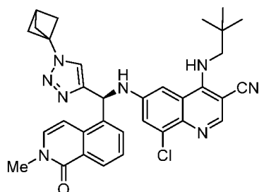
Verbindung 1
