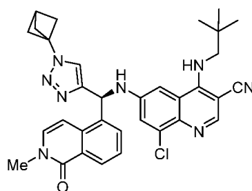
Verbindung 1
