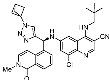
Composé 1.
