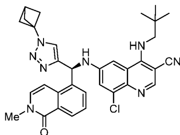
Composé 1.
