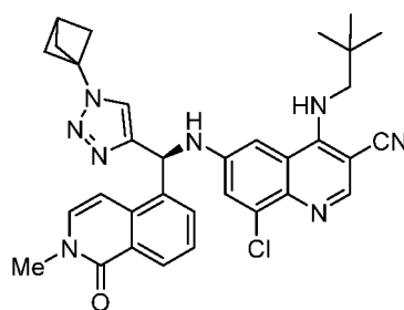
Verbindung 1
